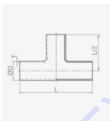
焊式等径三通 / Weld Equal Tee
