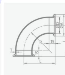
真空法兰式90°弯头 / KF 90° Elbow
