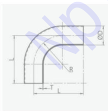
90°焊式长弯头 / 90° Weld Long Elbow
