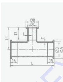
真空法兰式变径三通 / KF Reducer Tee
